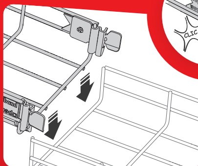
VERTICALE MONTAGE
